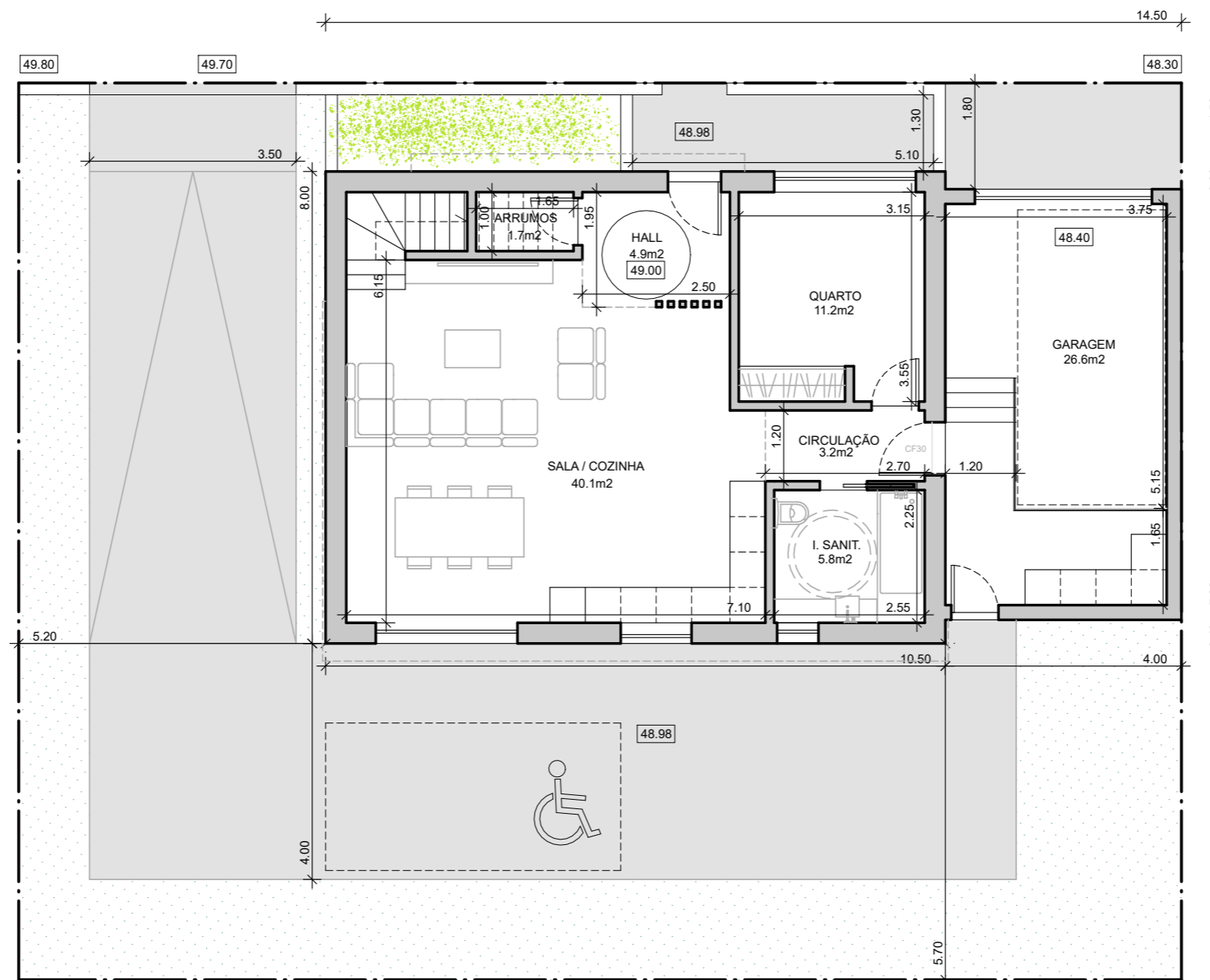
PLANTA PISO 0
